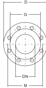
PN16 FLANGES
