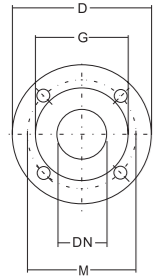
PN16 FLANGES
